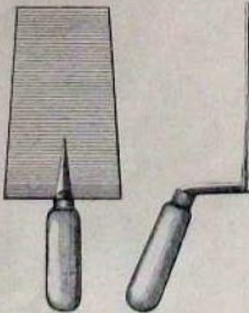
N o 154 de Maçon carrée de Lyon, de 12 o /m.
